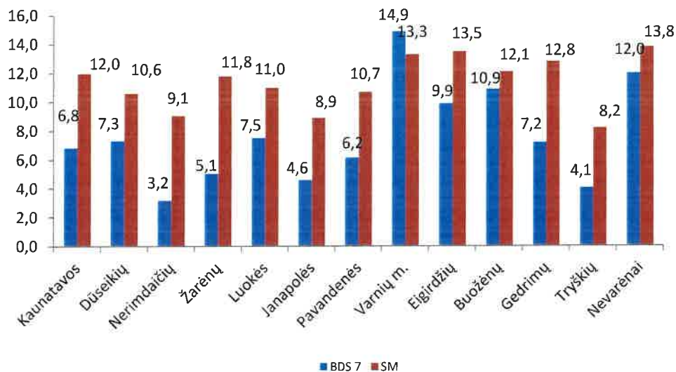
Išvalytų nuotekų kokybė gyvenviečių NVĮ 2022 metais, mg/l
